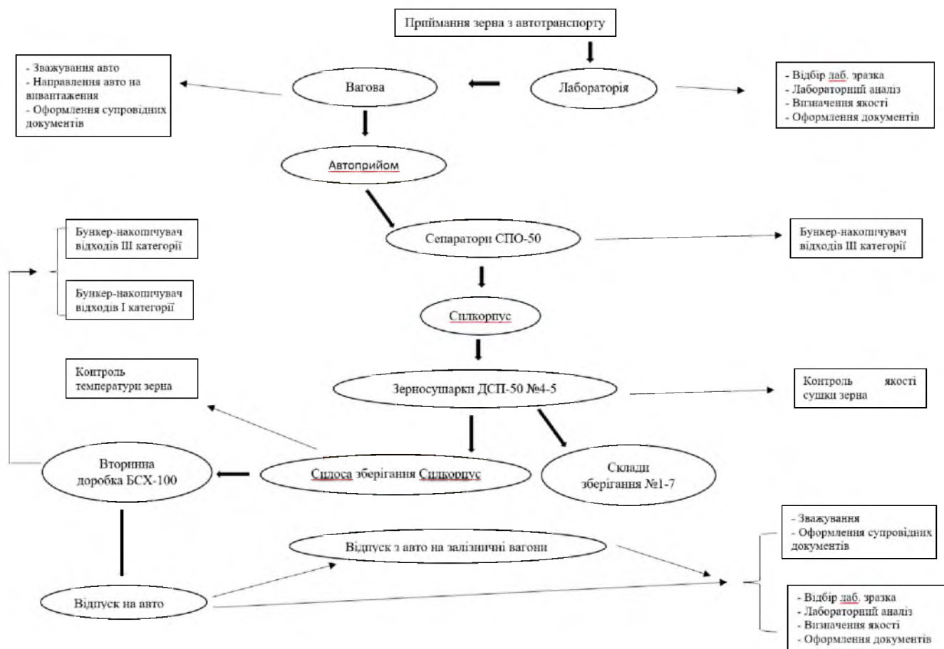
Рисунок 1.4 - Блок-схема виробничого процесу Елеватор №3
